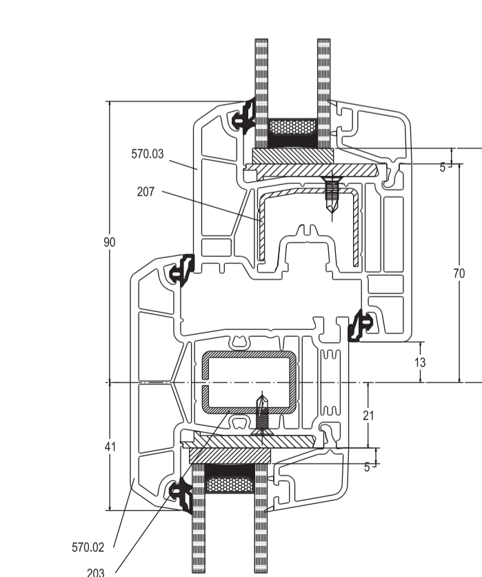
Комбинация - Глухое остекление импост/створка
